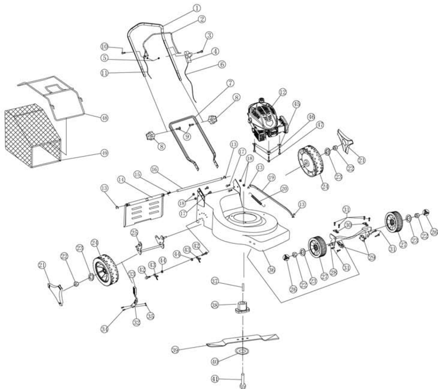
CT. C46S-B分解图
